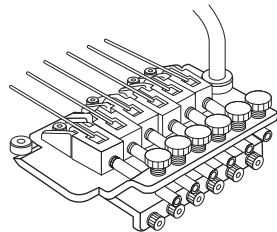
Chevalet Tremolo Verrouillé
