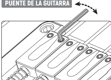
Ajuste de la altura de cuerda
